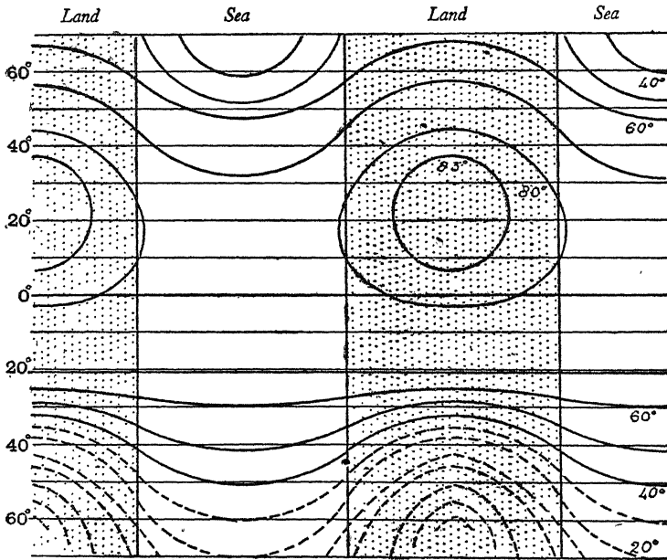
चित्र २६ : जुलाई के ताप के साधारण वितरण का रेखाचित्र
